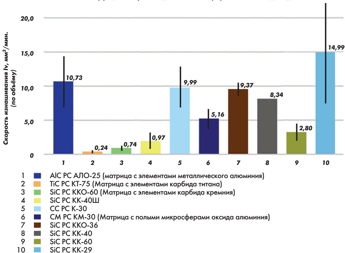
Рис. 5 Скорость изнашивания материалов
