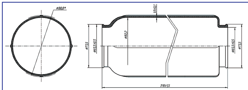
Диафрагма для УЭЦН "ODI" PP.041.06.0001 (аналог 9487)
