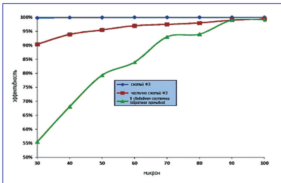
Эффективность фильтроэлементов из ППМ при сжатии
