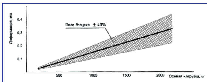
Диаграмма нагружения кольца демпфирующего
