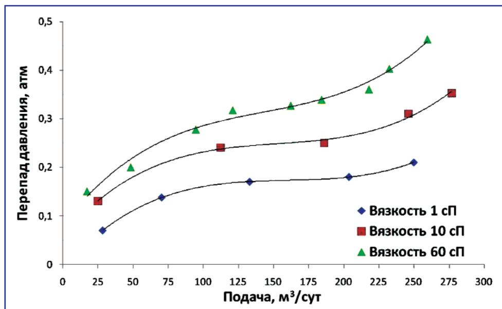
Расходно-перепадная характеристика для блока ФЭ из ППМ (14 шт.)
