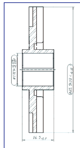
Рабочее колесо НОУ5-35.001-03
