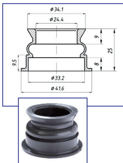
Сальфон ЕЮТИ.Г.566.001-Р к торцевому уплотнению 2Р25
