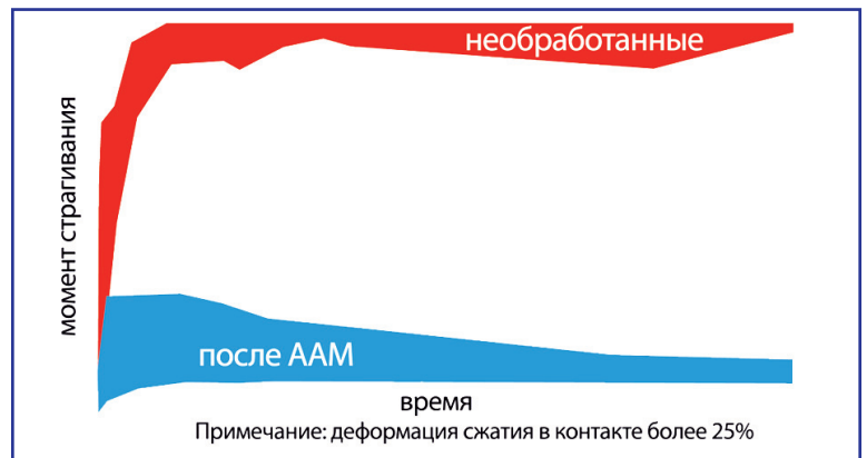
Результаты стендовых испытаний манжет необработанных и после адсорбционно-абсорбционной модификации в жидкой среде (материал - HNBR, твердость по Шор А - 87 ед. Шор-А)
