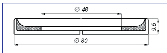
Прокладка РР.033.204.122 (ГН - 817.06.04)
