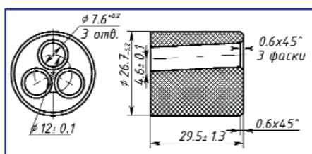
Уплотнитель КАБ.009
