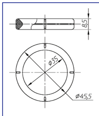
Вкладыш 180-3414069
