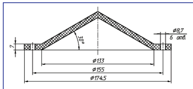
Уплотнитель PP.031.013.116
