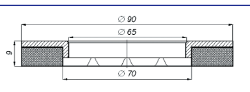
Подпятник обратный БЭП 01.250
