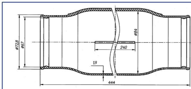
Диафрагма для УЭЦН "ODI" PP.041.06.0001 (аналог 9487)
