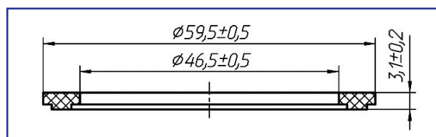
Уплотнение PP.031.011.117
