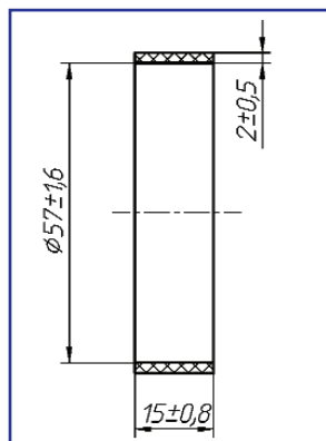
Кольцо 8ВЖ.214.990
