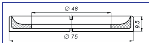
Прокладка ГН - 836.06.04
