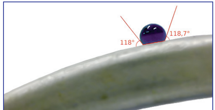
Краевой угол смачивания образца после испытаний на гидравлические характеристики
