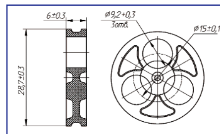
Уплотнитель РР.035.011.0028
