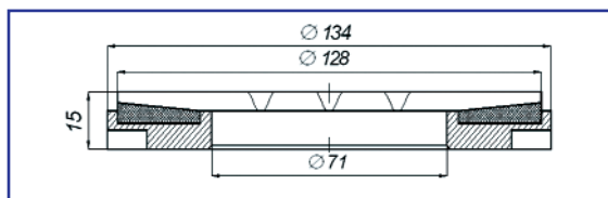
Подпятник БЭП 01.240 СБ
