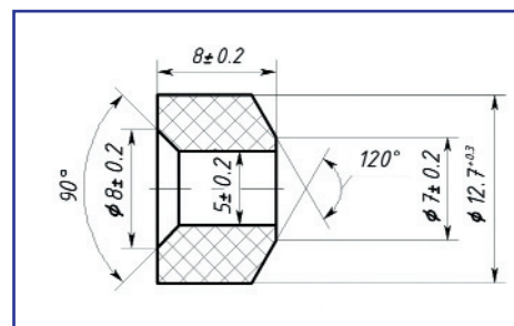
Седло ЕЮТИ.Г.390.144-Р
