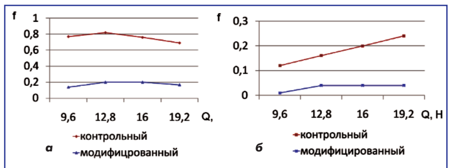
Зависимость коэффициента сухого трения f от нагрузки Q эластомерной композиции на основе БНКС-28 переходной вулканизации до и после ААМ в жидкой среде: а) при скорости 2,6 м/с; б) при скорости 6,2 м/с
