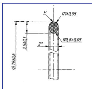
Кольцо каплевидное PP.031.108.183
