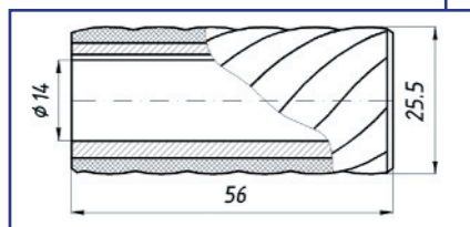
Втулка ЭП 028.03.03.000-01 СБ
