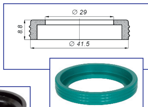
Манжета 1Н-21756 к торцевому уплотнению JOHN CRANE INT-0250-S-EPO
