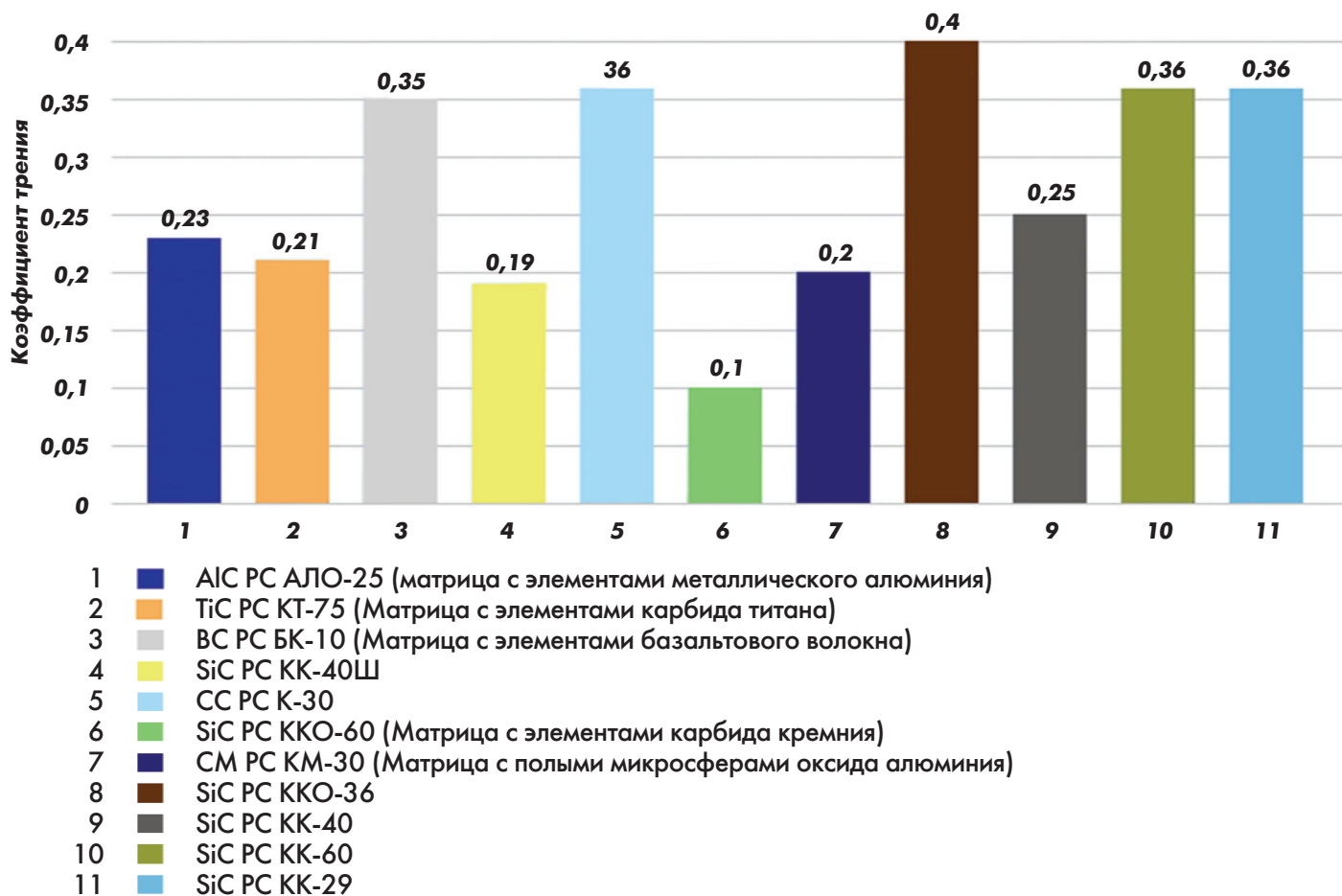
Рис. 4 Коэффициенты трения одноимённых пар трения по схеме диск-диск
