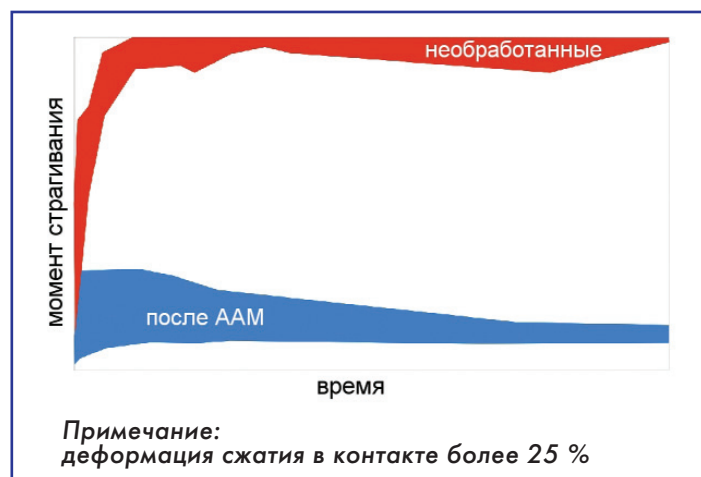
Результаты стендовых испытаний манжет необработанных и после адсорбционно-абсорбционной модификации в жидкой среде (материал - HNBR, твердость по Шор А - 87 ед. Шор А)
