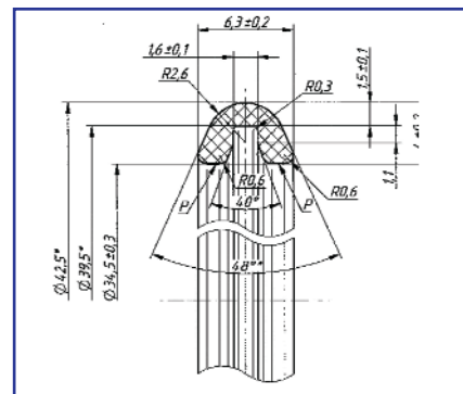
Кольцо Л-образное PP.031.109.184
