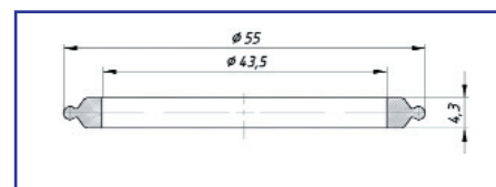
Кольцо Т-образное 46521402-450-43969
