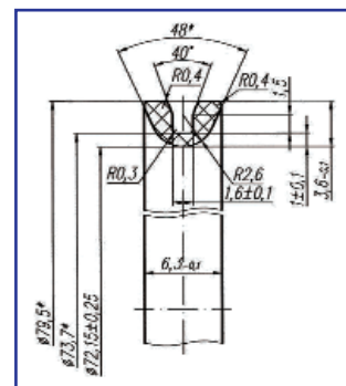
Кольцо V-образное PP.031.109.182
