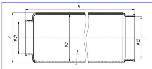
Диафрагма для УЭЦН "Centrilift" PP.041.006.05.357-01
