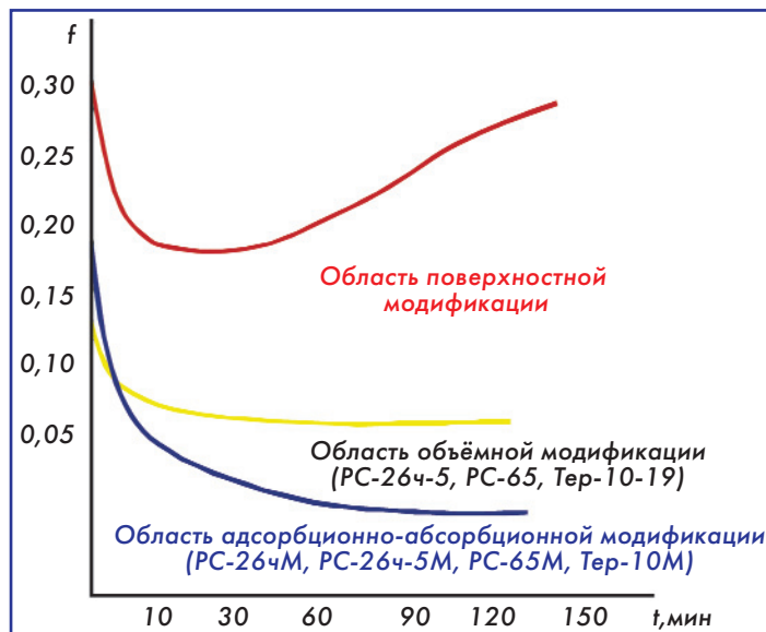
Результаты стендовых испытаний манжет необработанных и после адсорбционно-абсорбционной модификации в жидкой среде (материал - HNBR, твердость по Шор А - 87 ед. Шор А)
