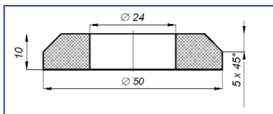
Отбойник PP.031.204.121 на вал 2ПБ 92.00.004
