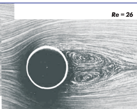
Картина обтекания цилиндрического тела (фото Sadatoshi Taneda)
