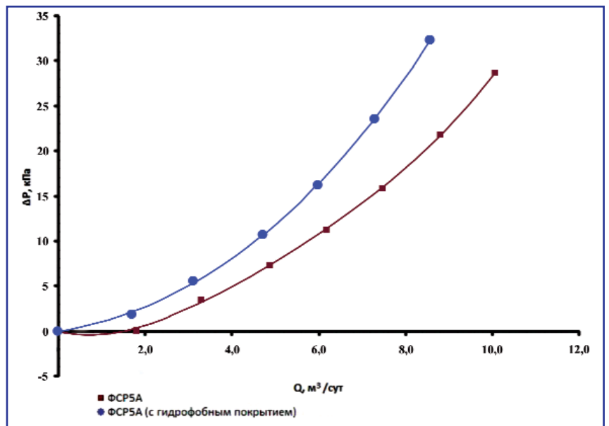
Сравнительная расходно-перепадная характеристика фильтроэлементов ФСП 105х95х35-200 (ФСП5А)
