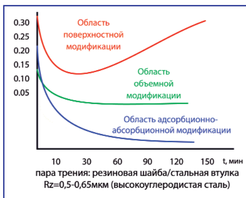
Зависимость коэффициента трения f от времени t для эластомерных композиций, модифицированных различными методами
