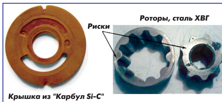
Рис. 6,6 Испытания в лаборатории "ЛЕПСЕ-Нефтемаша" на абразивную стойкость неподвижных крышек этого насоса, изготовленные из композиции "КАРБУЛ Si-C", взаимодействующих с внутренними роторами из традиционных высокопрочных сталей показали - износа, эквивалентного металлу, у крышек из композиции "КАРБУЛ Si-C" не наблюдается
