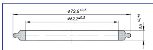
Кольцо Т-образное PP.041A.04.63 для подшипника серии 544
