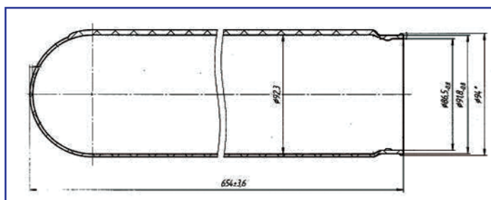
Диафрагма PP.031.006.368
