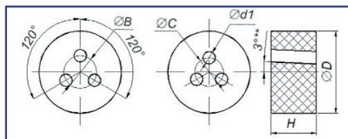
Тройник ТМГ ДМ 03.06
