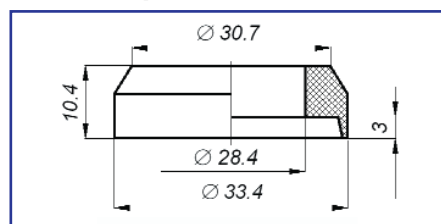
Отбойник на вал 7/8" гидрозащиты ГЗ.004
