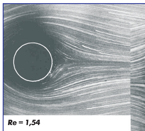
Картина обтекания цилиндрического тела (фото Sadatoshi Taneda)
