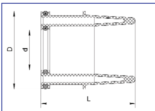
Протектор поршня поршневой гидрозащиты
