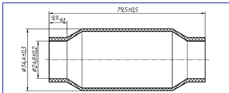
Компенсатор АКШ-43/PP.033.006-110
