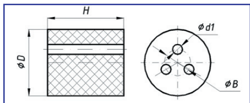
Вставка ТМГ ДМ 03.05
