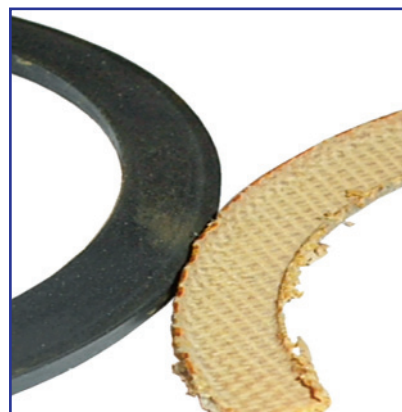
Внешний вид шайб из эластомерного композита К-38 ООО "РЕАМ-РТИ" (слева) и текстолита (справа) после указанных испытаний
