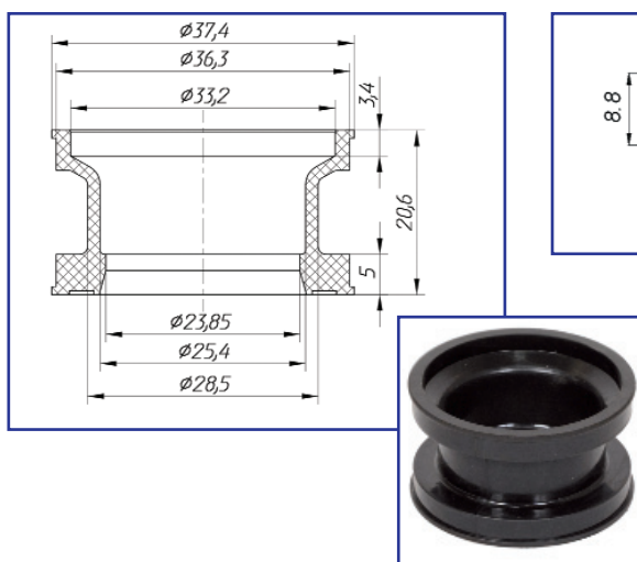
Сальфон к торцевому уплотнению JOHN CRANE INT-0250-S-EPO
