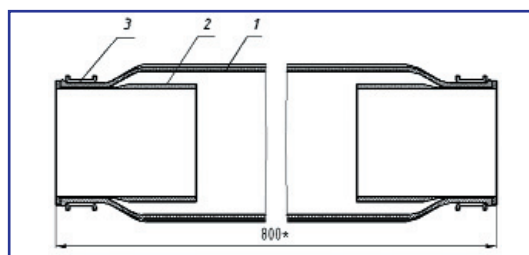
Комплект РТИ для диафрагм гидрозащиты в сборе РР.033.202.034, РР.033.202.035:
