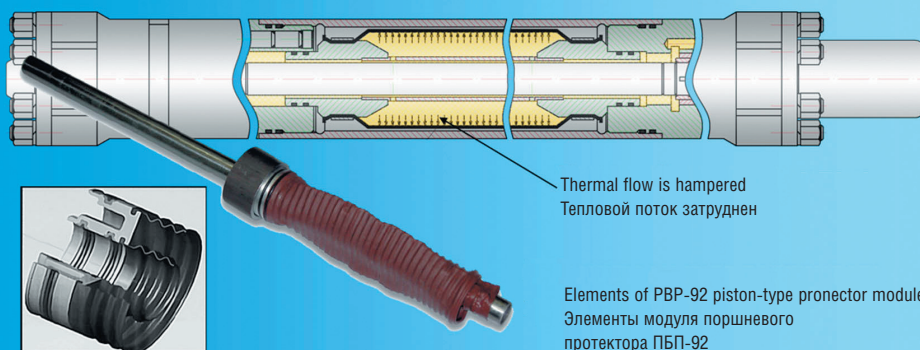
PB-92 Diaphragm-type protector module / Модуль диафрагменный протектора ПБ-92
